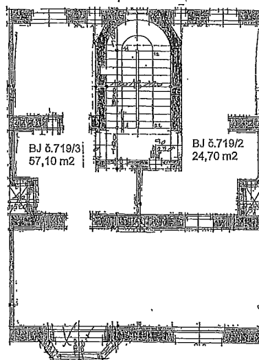
2. nadzemní podlaží
