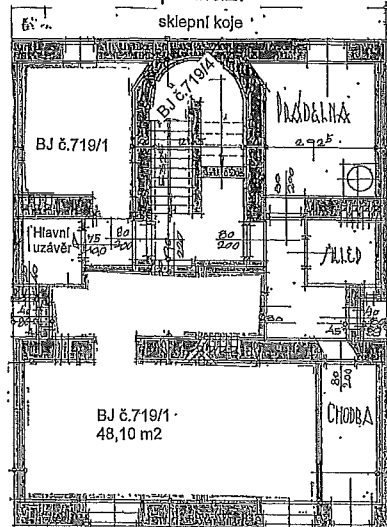
1. nadzemní podlaží
